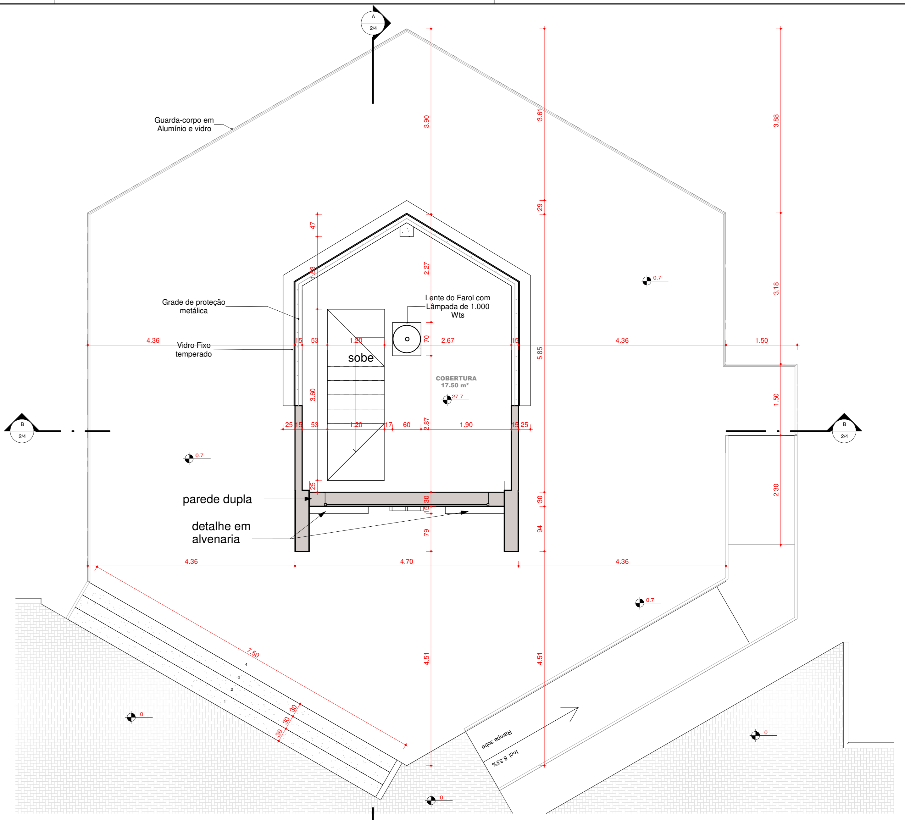
1 10 - PISO COBERTURA 1 : 50
