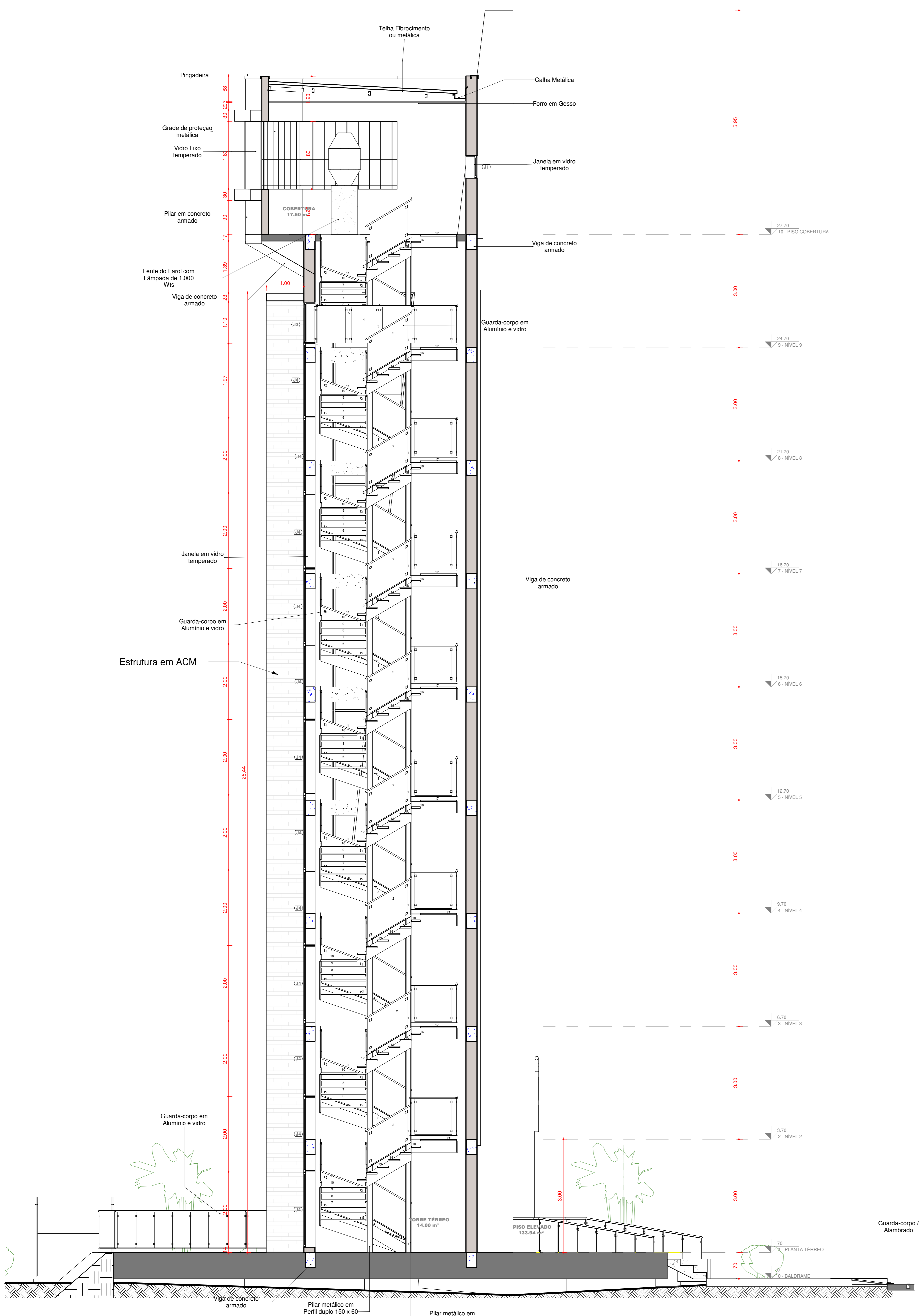
A Corte AA 1 : 50
